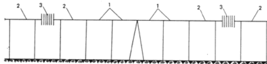
Схема прокладки трубопровода на опорах
