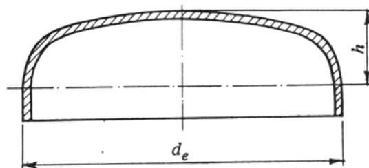
Черт. 3. Заглушка эллиптическая
