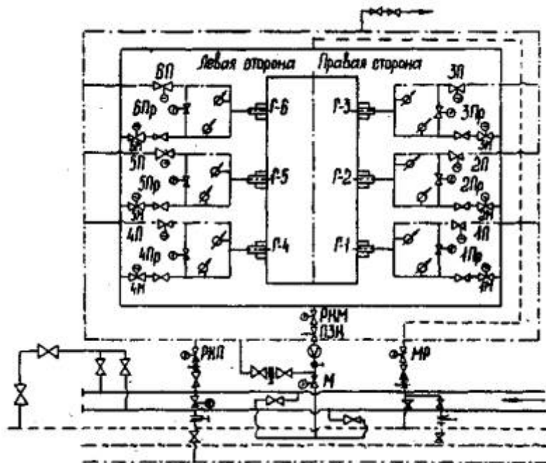
Рис. 2. Схема паромазутопроводов котла КВГМ-180:
