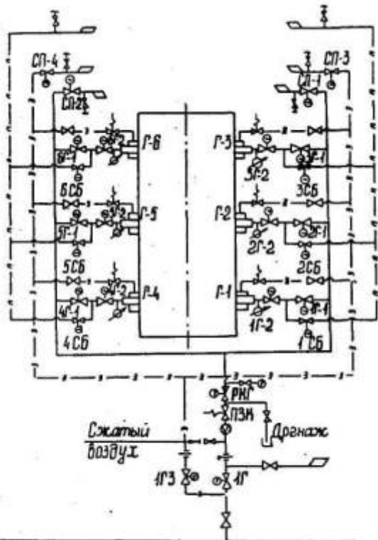
Рис. 3. Схема газопроводов котла КВГМ-180:
